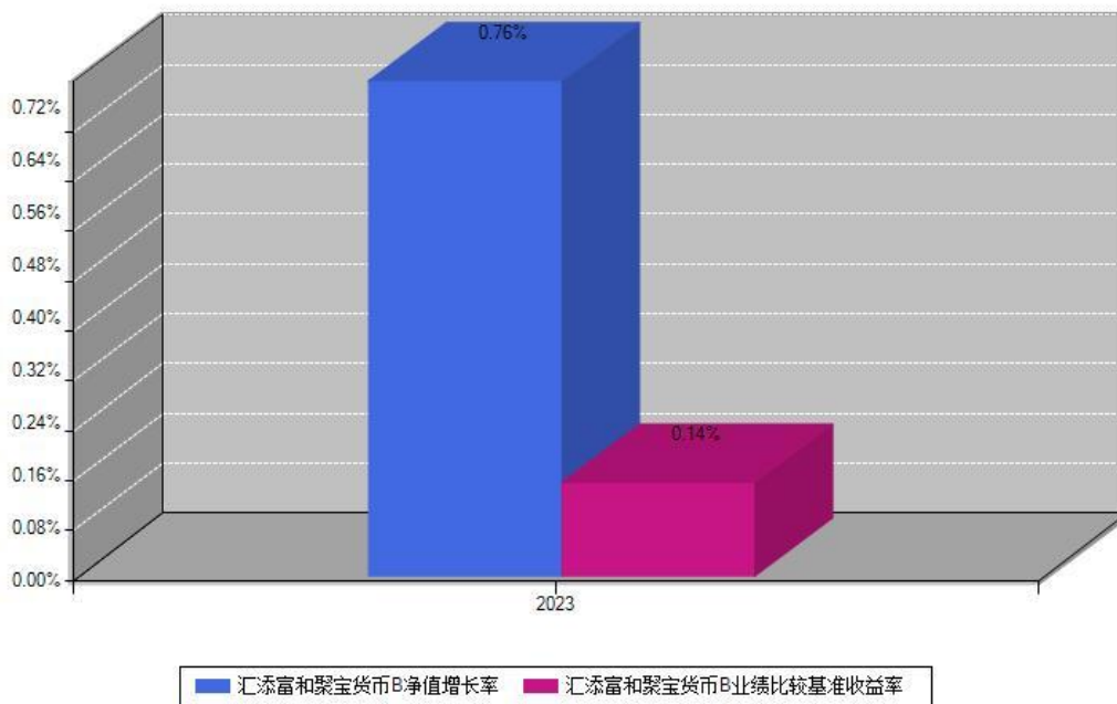
汇添富和聚宝货币B每年净值增长率与同期业绩基准收益率对比图
