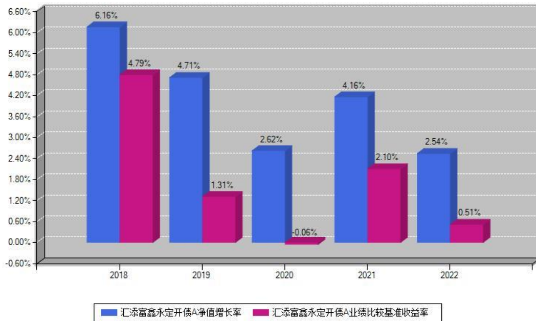
汇添富鑫永定开债A每年净值增长率与同期业绩比较基准收益率对比图
